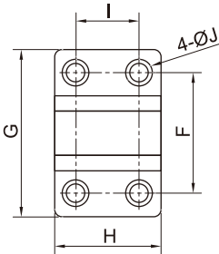
四孔安装座
